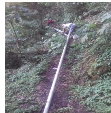
LIMPIA, TRAZO, NIVELACIÓN Y COLOCACIÓN DE TUBERÍA DE Fo.Go. DE 3" DE DIÁMETRO
