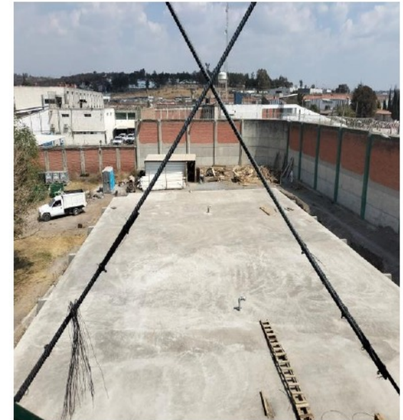
TANQUE CISTERNA CON CAPACIDAD DE 1500 M3
