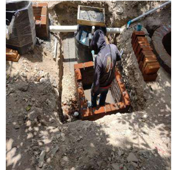
INSTALACIÓN DE BIODIGESTOR, CONSTRUCCIÓN DE REGISTROS DE INSPECCIÓN
