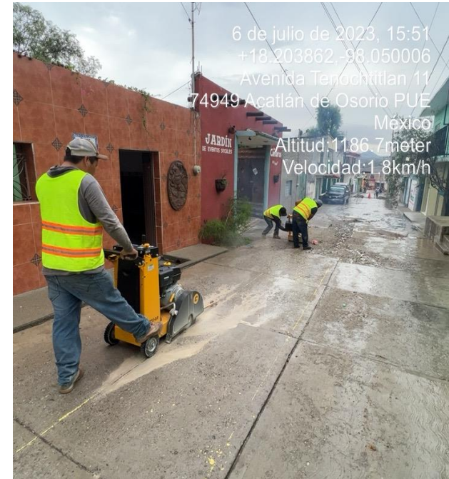
CORTE EN PAVIMENTO DE CONCRETO HIDRÁULICO
