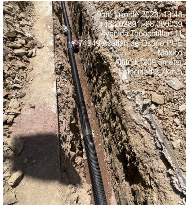
INSTALACIÓN DE TUBERÍA
